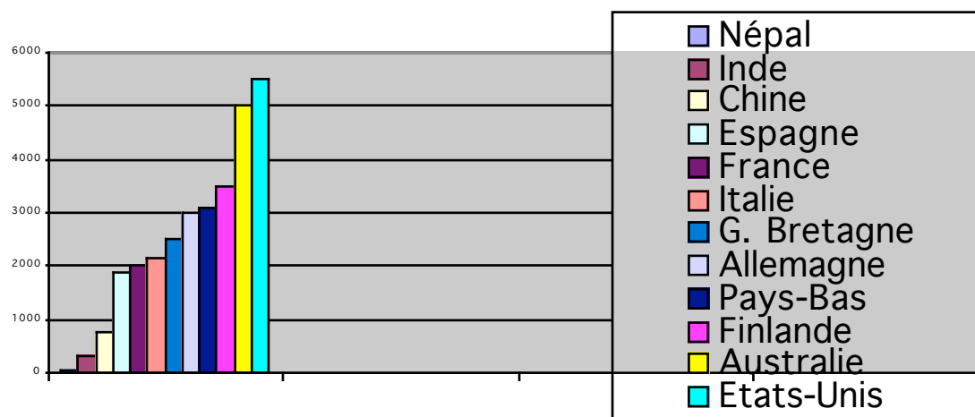
Graphique 2 Émission d'équivalent-carbone en 1998 (en kg par habitant)
